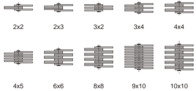
链板组合 Plate lacing
